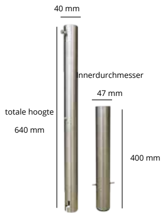
Bodenanker
